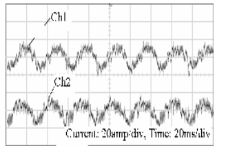
Fig.26.Ch1: i_{s\_a1} Ch2: i_{s\_a2}
